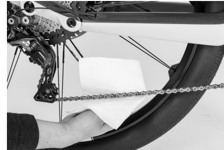
Abb. 21: Kette schmieren
